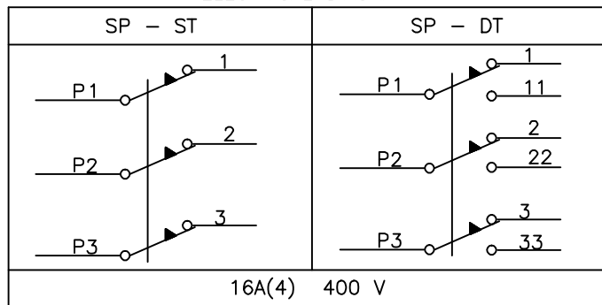
SCHEMA ELETTRICO ELECTRICAL DIAGRAM :
